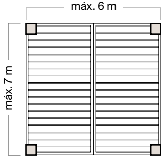
Módulo doble Sin poste central
