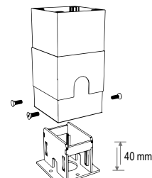
Pie nivelador (150x150 mm)
