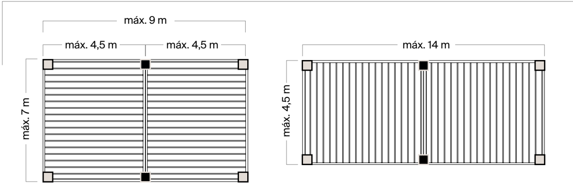
2 módulos sencillos Con postes compartidos
